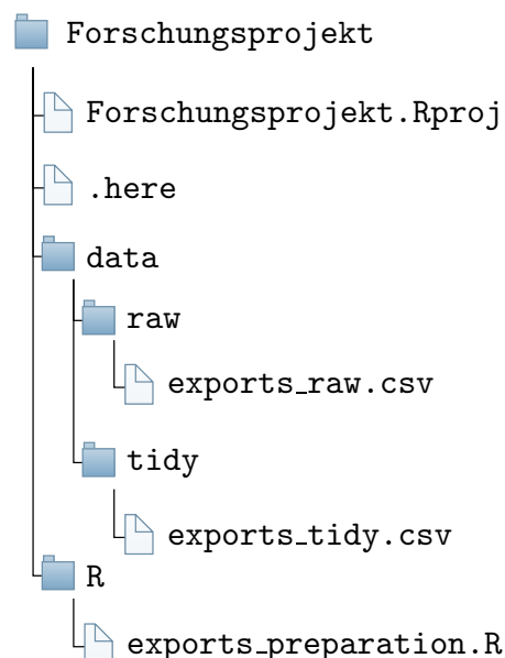
Abbildung 4.4: Eine übersichtliche Art und Weise Ihre Daten zu speichern. Die Dateien im Unterordner 'raw' werden nie geändert. Die Datei 'exports-tidy' im Ordner 'tidy' wurde mit dem Skript 'exports-preparation.R' aus dem Rohdatensatz 'exports-raw.csv' erstellt.
