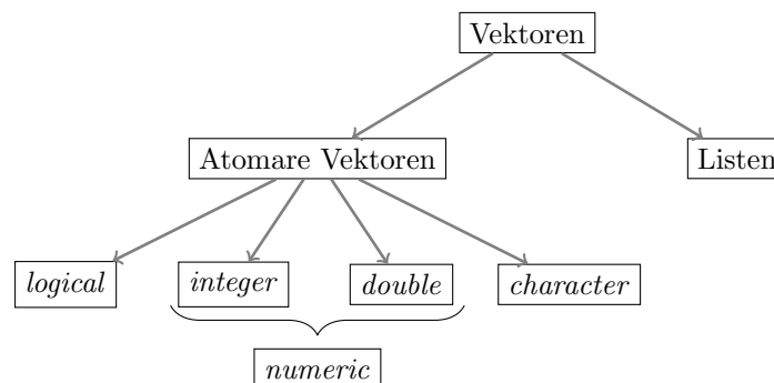
Abbildung 3.1: Arten von Vektoren in R
