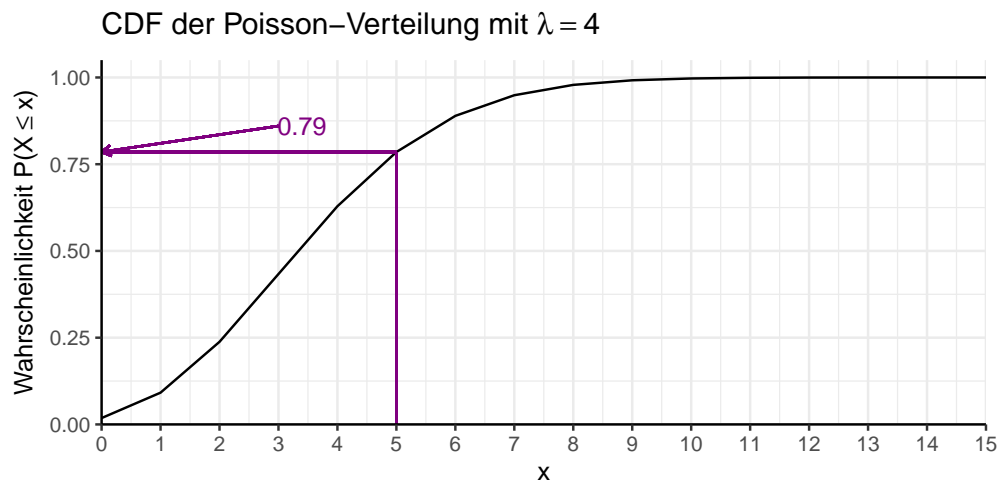
Abbildung 7.9: Kumulierte Wahrscheinlichkeitsfunktion der Poisson-Verteilung mit \lambda = 4
