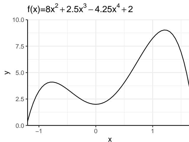
Abbildung 6.6: Graph der zu optimierenden Funktion.
