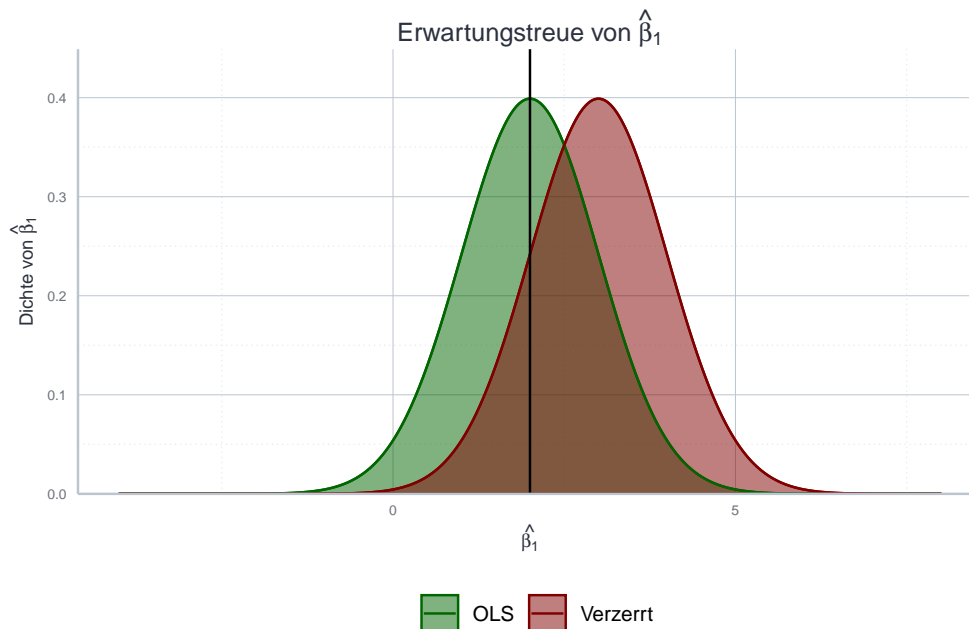
Abbildung 11.3: Erwartungstreue von \hat{\beta} unter Annahmen 1 bis 3.
