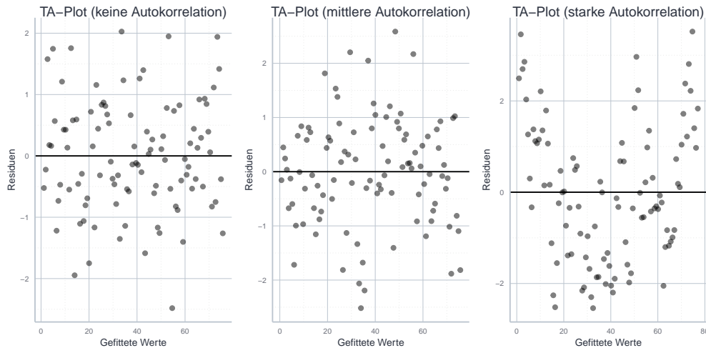
Abbildung 11.10: Unterschiedlich starke Autokorrelation im Tukey-Anscombe Plot.
