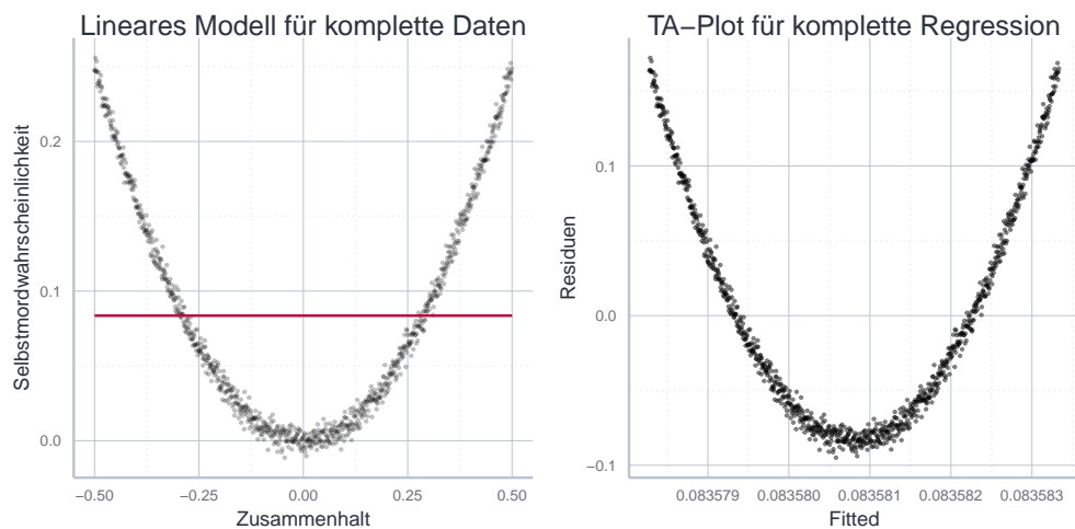
Abbildung 11.17: Die Schätzung eines linearen Modells auf die simulierten Durkheim-Daten ist eindeutig fehlspezifiziert.
