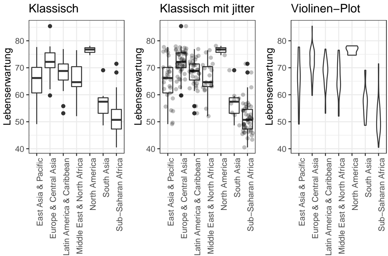
Abbildung 6.18: Vergleich von klassischen Darstellungen und dem Violinenplot
