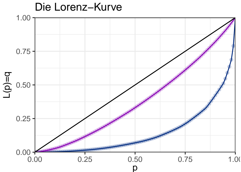
Abbildung 6.10: Vergleich zweier Lorenz-Kurven
