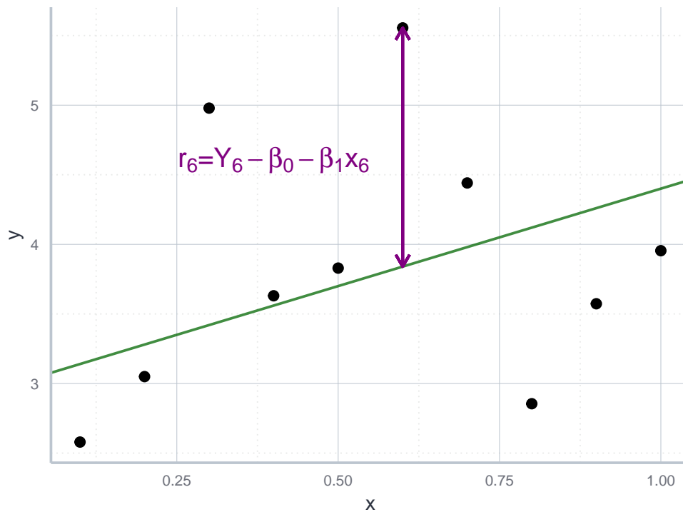
Abbildung 10.1: OLS Gerade als jene Gerade, welche den Abstand zu den quadrierten Residuen minimiert.
