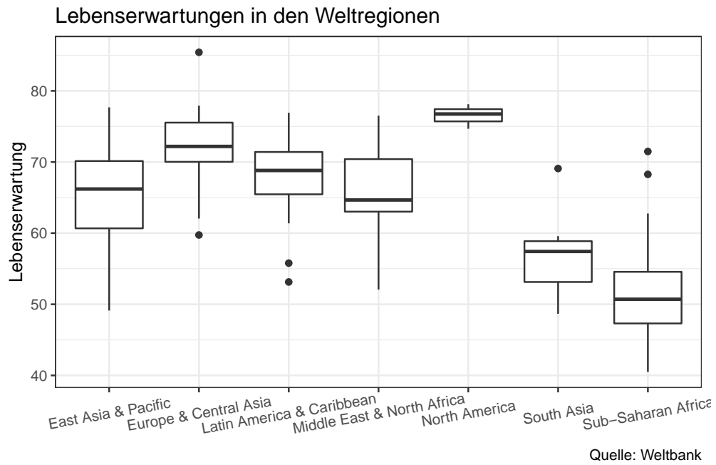
Abbildung 6.16: Darstellung der Lebenserwartungen in den Weltregionen anhand eines Boxplots
