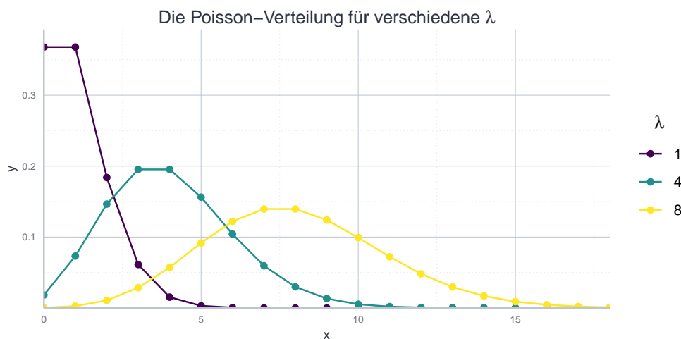
Abbildung 7.7: Poisson-Verteilung für verschiedene Parameter.
