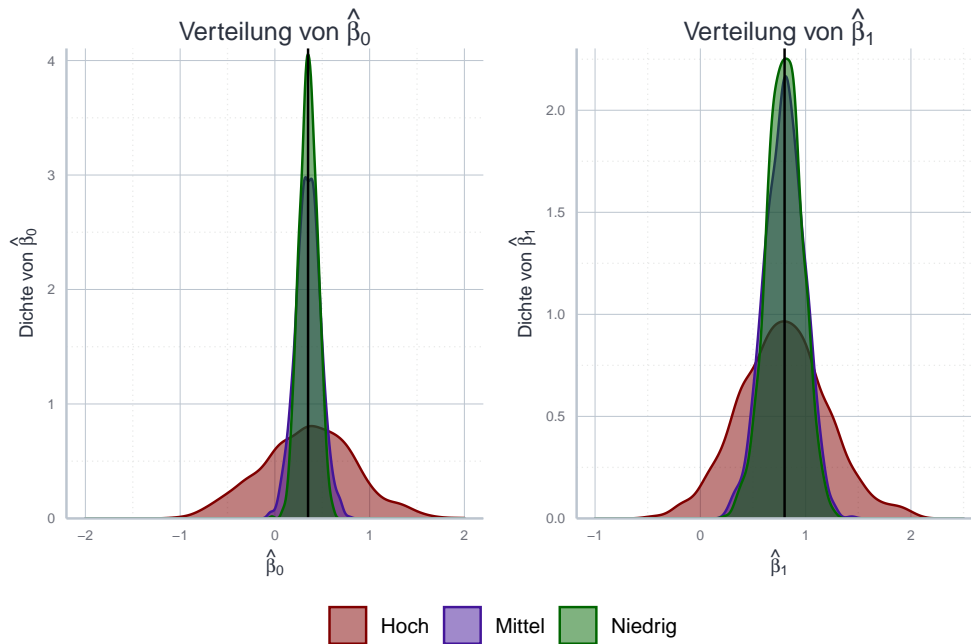
Abbildung 11.8: Folgen der Autokorrelation mit Bezug auf Erwartungstreue und Effizienz anhand von Monte Carlo Simulationen.
