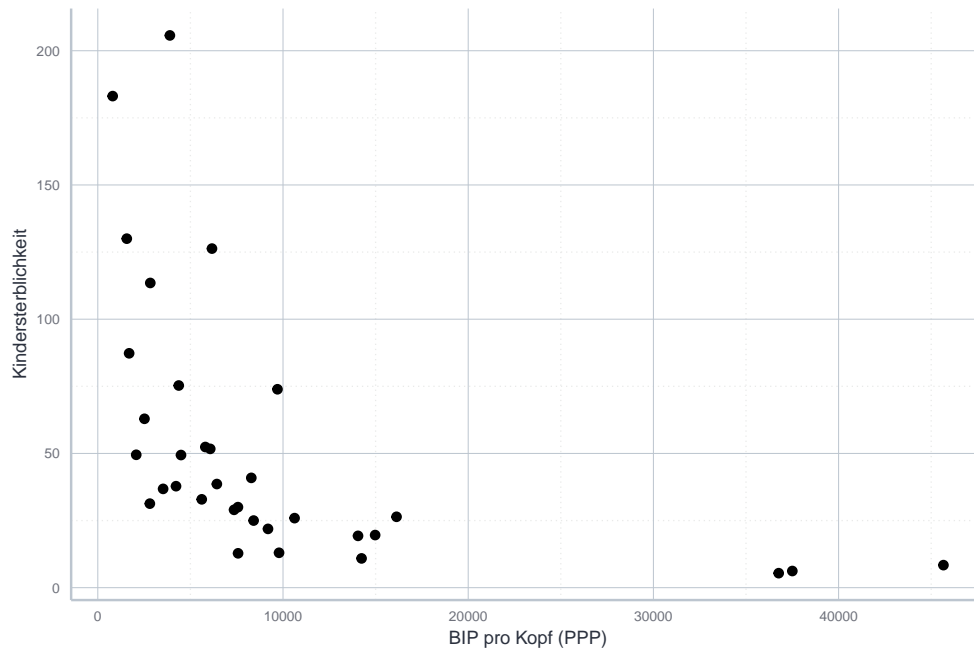
Abbildung 11.14: Nicht-linearer Zusammenhang zwischen BIP und Kindersterblichkeit.
