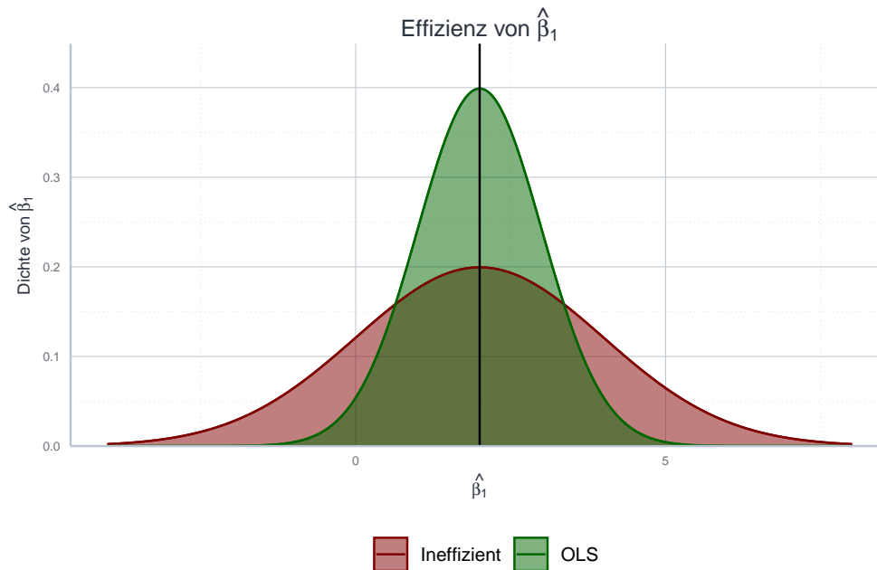
Abbildung 11.4: Effizienz von \hat{\beta} unter Annahmen 1 bis 4.
