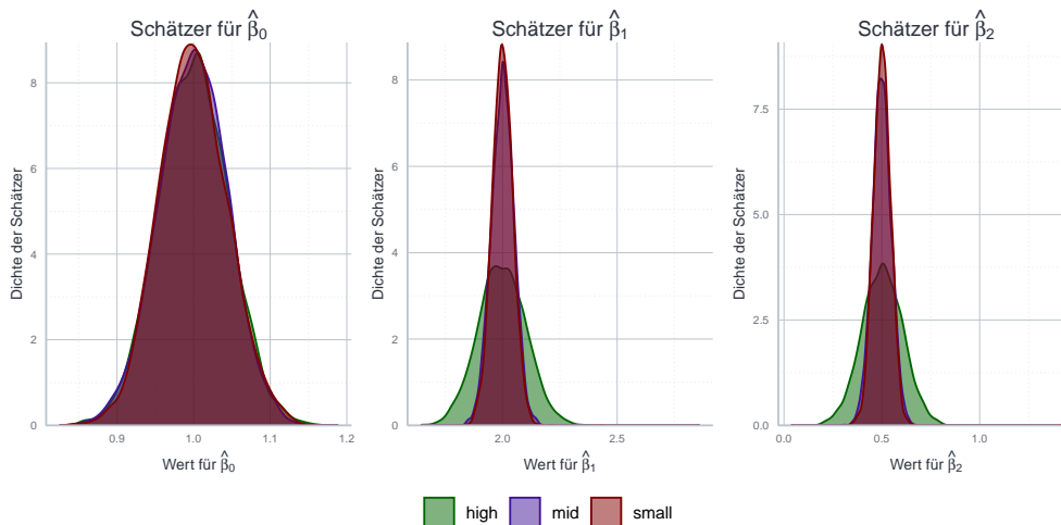
Abbildung 11.11: Folgen der Multikollinearität mit Bezug auf Erwartungstreue und Effizienz anhand von Monte Carlo Simulationen.
