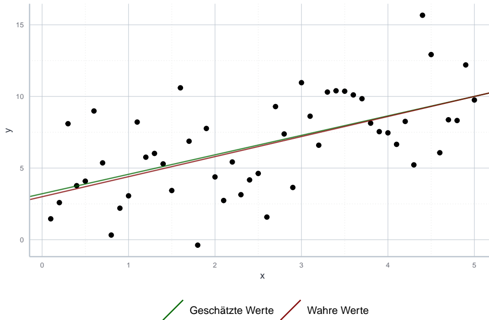
Abbildung 10.7: Vergleich der geschätzten und wahren Gerade unserer Stichprobe.
