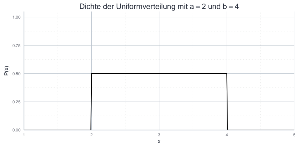
Abbildung 7.12: Dichte der Uniformverteilung mit a = 2 und b = 4
