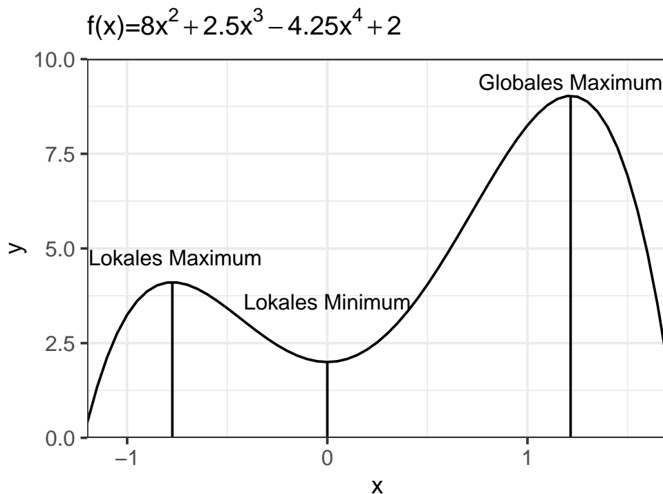
Abbildung 6.4: Beispiel für Extremwerte
