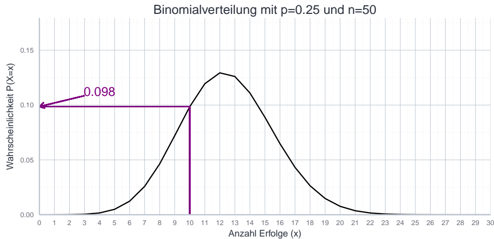
Abbildung 7.2: Beispiel einer Binomialverteilung mit p=0.25 und n=50 .
