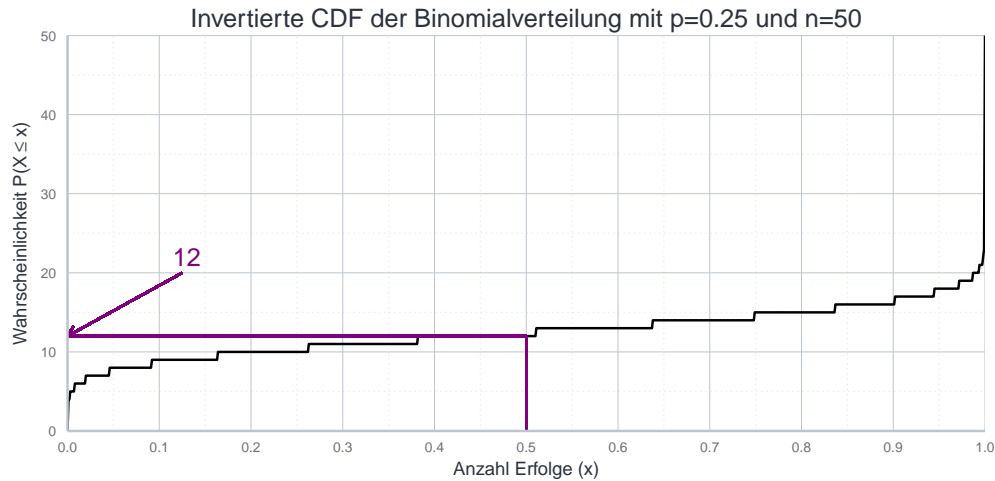
Abbildung 7.4: Graph der invertierten kumulierten Wahrscheinlichkeitsfunktion der Binomialverteilung mit p = 0.25 und n = 50
