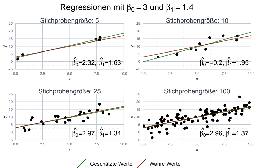
Abbildung 10.8: Vergleich der geschätzten Parameterwerte mit den wahren Werten unter verschiedenen Stichprobengrößen.
