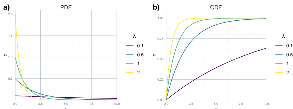
Abbildung 7.15: Beispielhafter Vergleich einer PDF und CDF bei Exponentialverteilung
