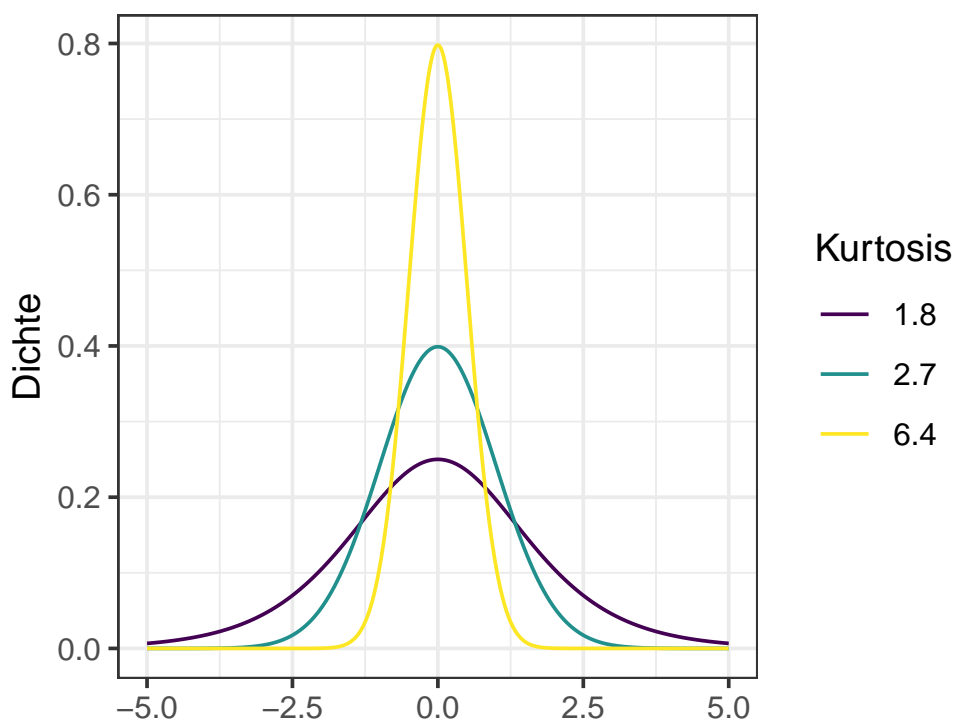
Abbildung 6.14: Beispiel von Verteilungen mit verschiedener Kurtosis
