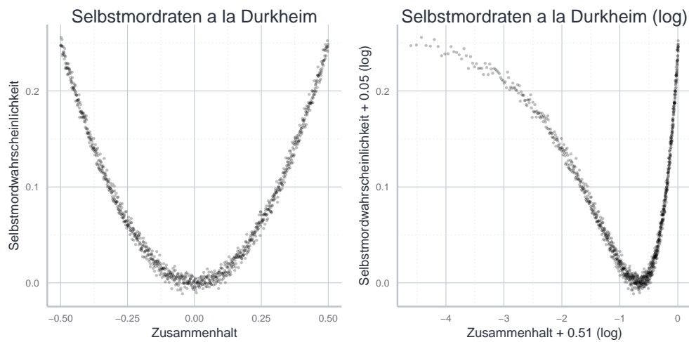
Abbildung 11.16: Simulierte Daten für Durkheim-Beispiel zum Zusammenhang zwischen sozialem Zusammenhalt und der Wahrscheinlichkeit zum Selbstmord.
