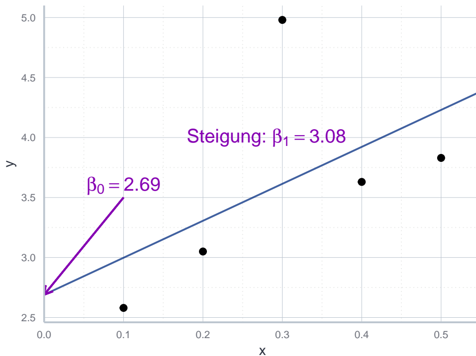
Abbildung 10.2: Regressionsgerade mit den berechneten Parameterwerten.
