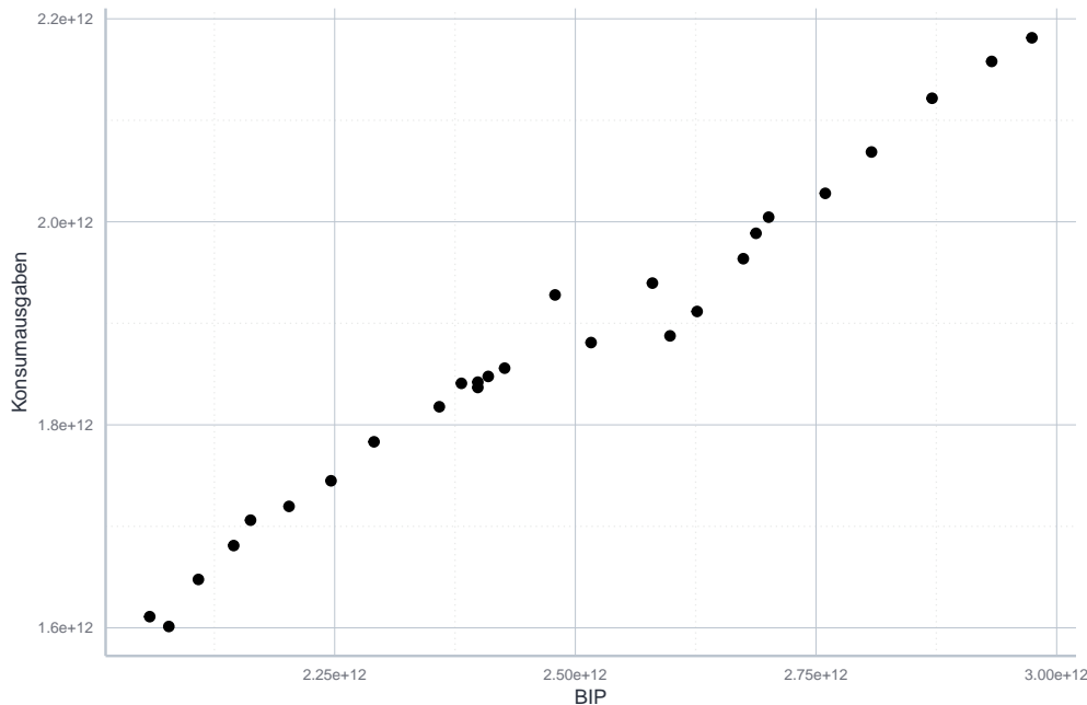
Abbildung 11.13: Linearer Zusammenhang zwischen BIP und Konsumausgaben.
