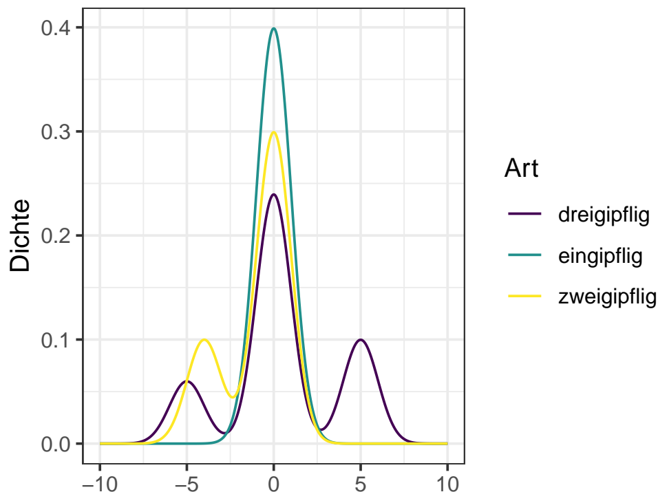
Abbildung 6.11: Beispiele multimodaler Verteilungen
