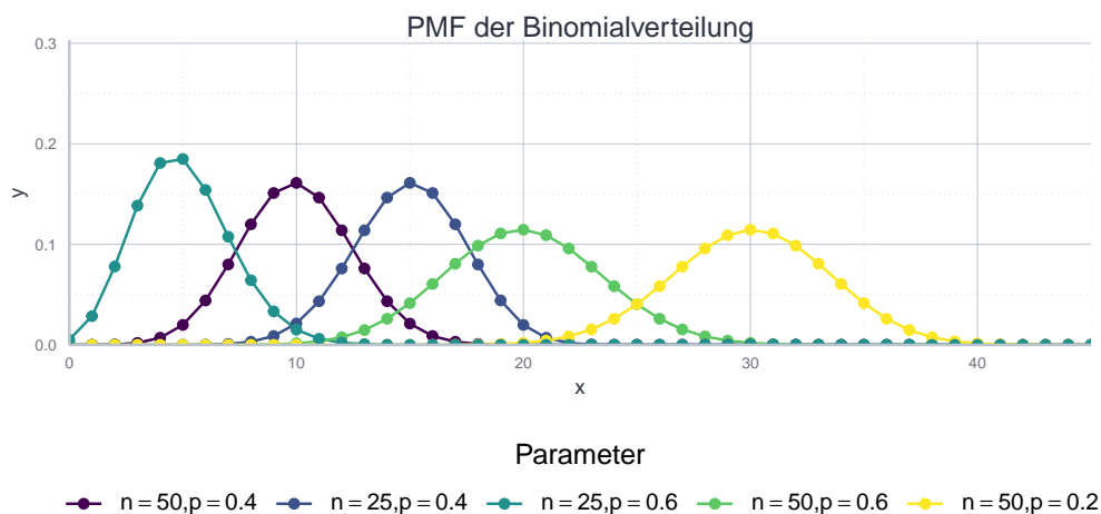
Abbildung 7.1: Die Wahrscheinlichkeitsverteilung der Binomialverteilung für verschiedene Parameterwerte.
