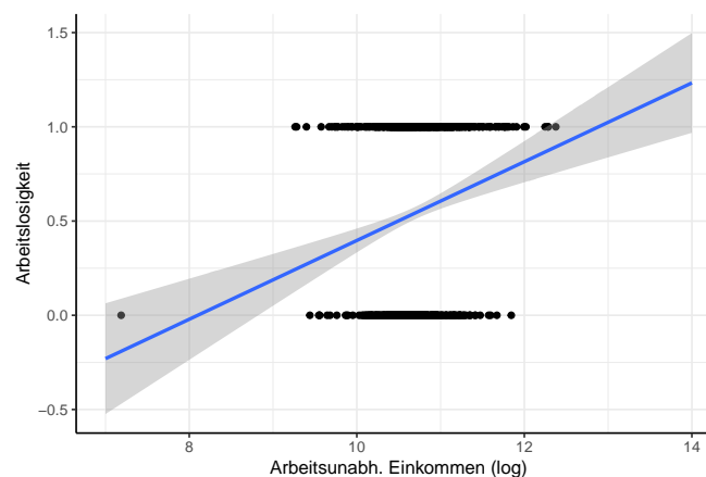
Abbildung 12.1: Schätzung mit OLS Modell.
