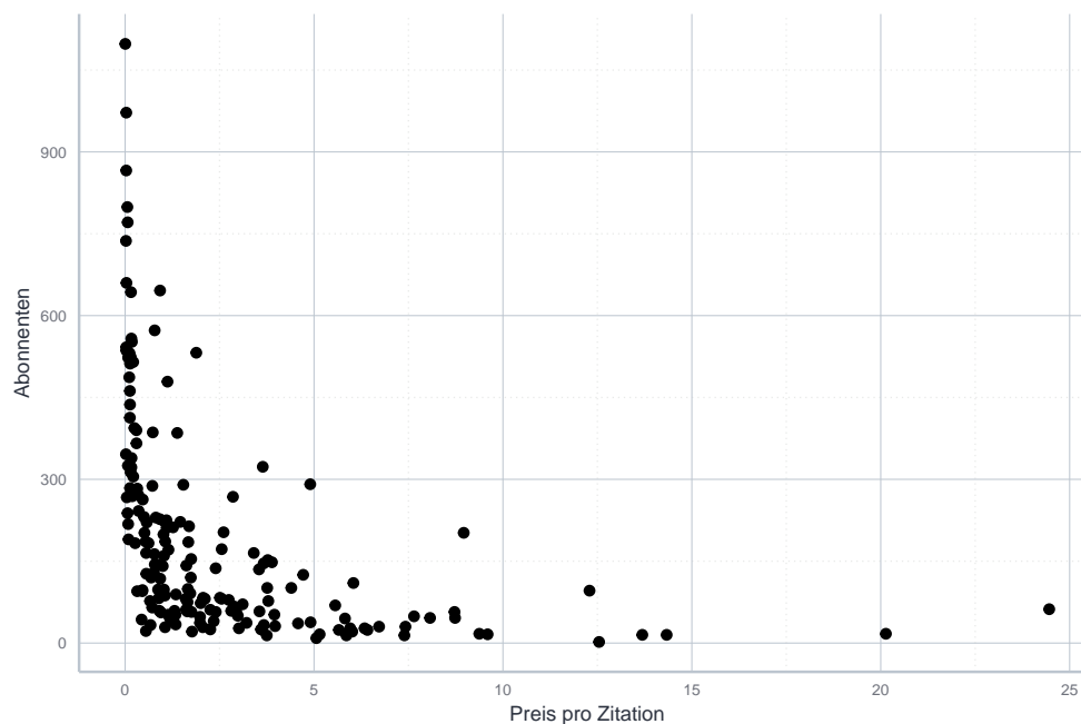
Abbildung 11.20: Nicht-linearer Zusammenhang zwischen Abonnenten und dem Preis pro Zitation
