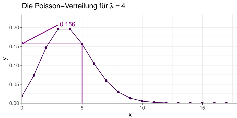
Abbildung 7.8: Poisson-Verteilung mit ausgewählten Parameterwerten.
