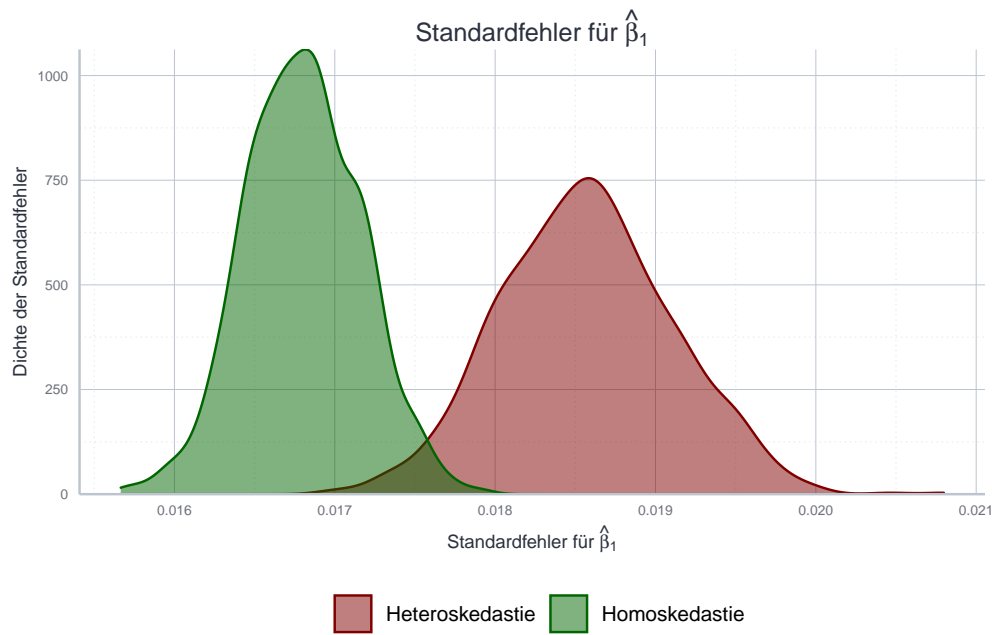
Abbildung 11.6: Vergleich der Standardfehler von \hat{\beta} bei Homoskedastie und Heteroskedastie.
