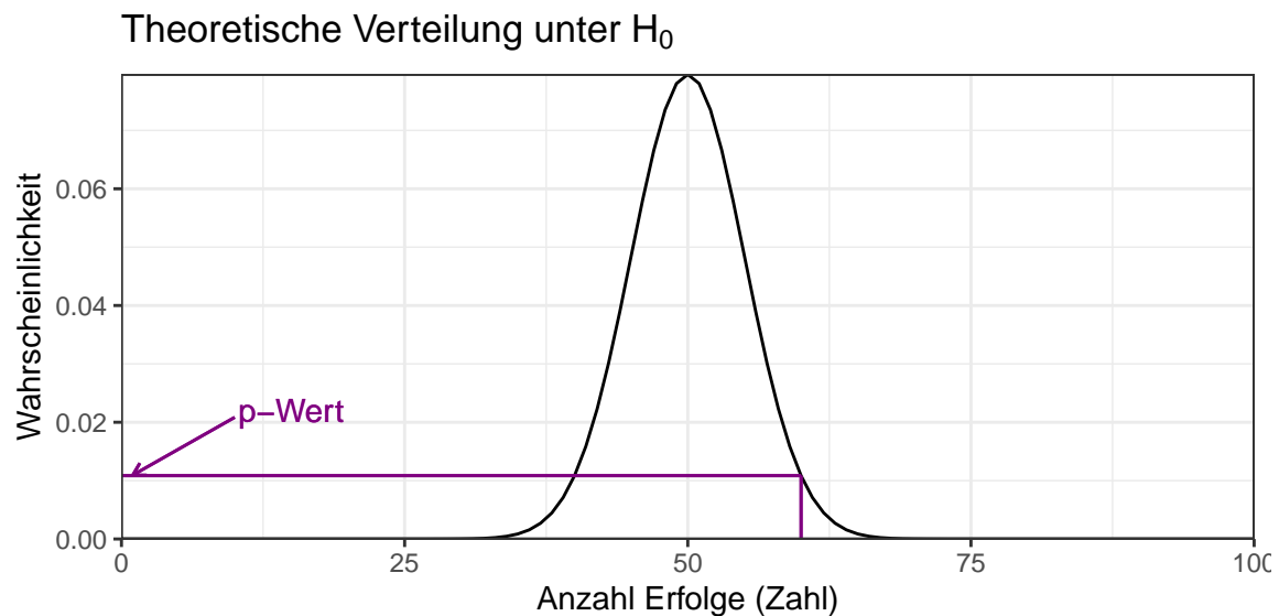
Abbildung 9.3: Ablesen des p-Werts aus der theoretischen Verteilung.
