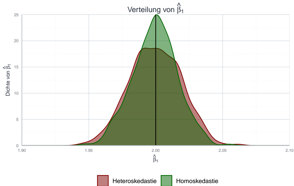
Abbildung 11.5: Vergleich der Verteilung der mit Monte Carlo geschätzten Werte für \beta_1 mit dem wahren Wert.
