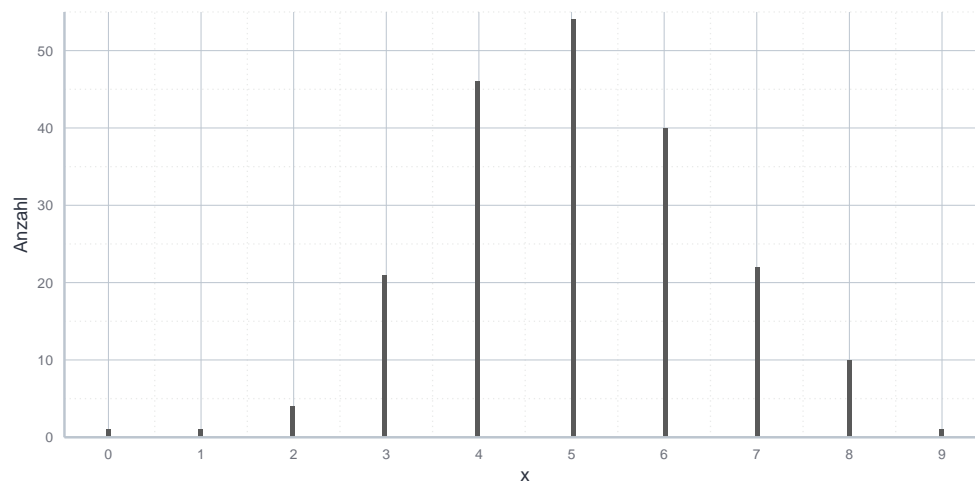
Abbildung 7.5: Histogram für einen Münzwurf.
