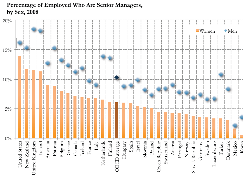
Abbildung 5.3: Beispiel für einen ‘unbalancierten’ Plot
