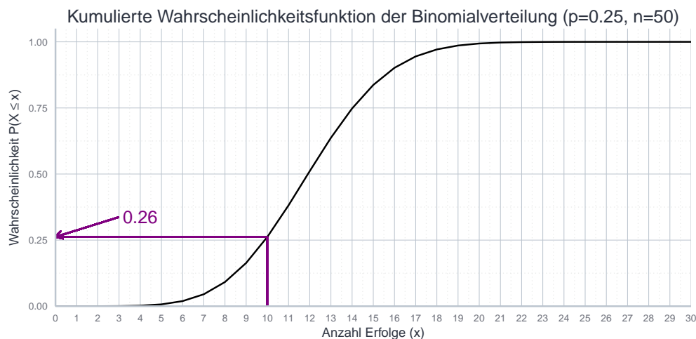
Abbildung 7.3: Kumulative Wahrscheinlichkeitsfunktion mit p=0.25 und n=50
