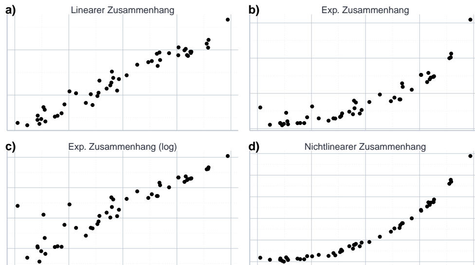
Abbildung 11.1: Lineare und nichtlineare Zusammenhänge.
