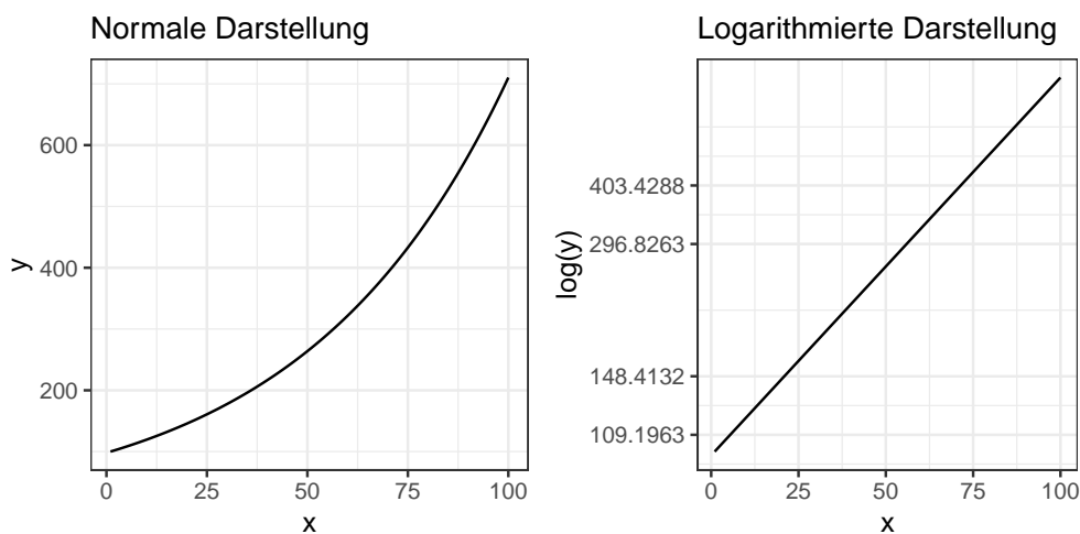
Abbildung 6.1: Vergleich normaler und logarithmierter Darstellung
