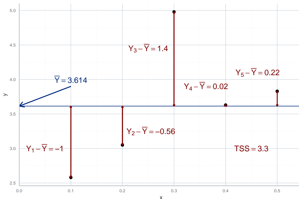
Abbildung 10.3: Werte für die Summe der totalen Abweichungen (TSS).
