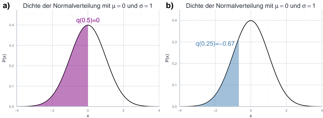
Abbildung 7.11: Vergleich des 0.25- und 0.5-Quantils
