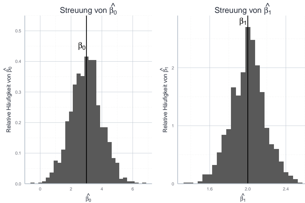
Abbildung 10.6: Vergleich der Effizienz zweier Schätzer über ihre jeweilige Streuung.
