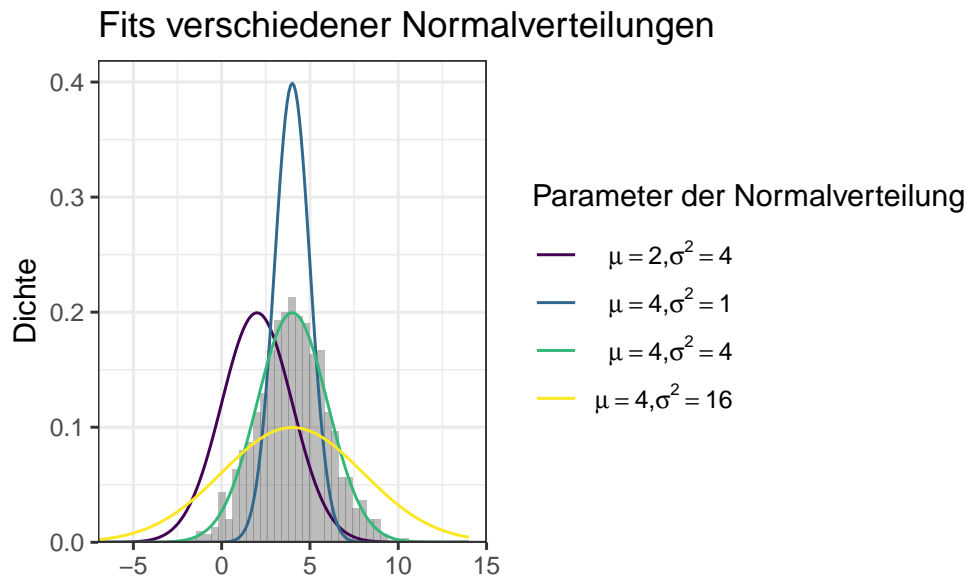
Abbildung 6.9: Beispiel zur Verdeutlichung von Fits verschiedener Normalverteilungen mit unterschiedlichen Parameterwerten
