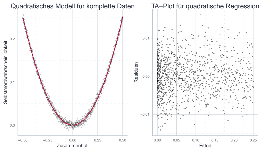
Abbildung 11.19: Durch das Hinzufügen eines quadratischen Terms in die Schätzgleichung kann das Modell korrekt spezifiziert und geschätzt werden.
