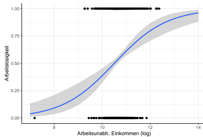
Abbildung 12.2: Funktionaler Zusammenhang, den ein binäres Modell abbilden sollte.
