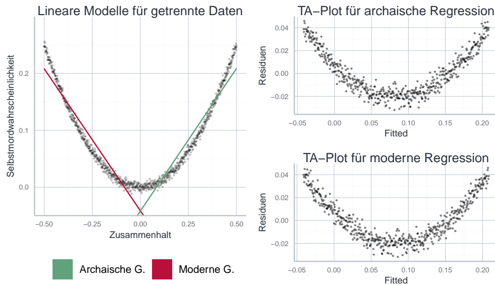
Abbildung 11.18: Auch eine Aufspaltung der Samples führt nicht dazu, dass der nicht-lineare Zusammenhang richtig geschätzt wird.
