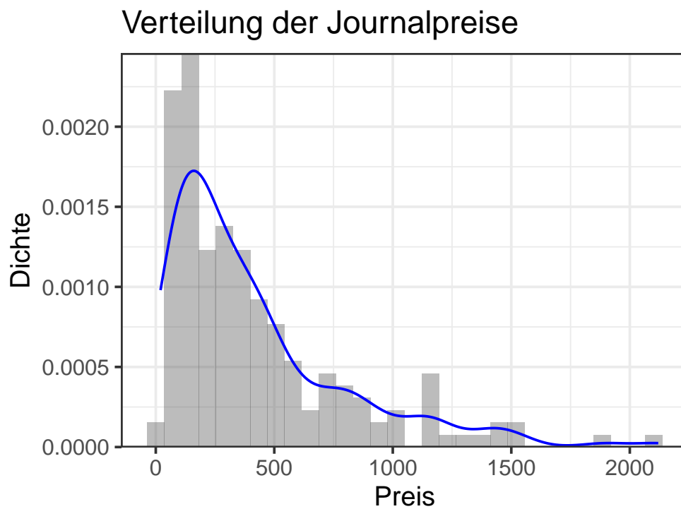
Abbildung 6.13: Rechts-schiefe Verteilung der Journalpreise
