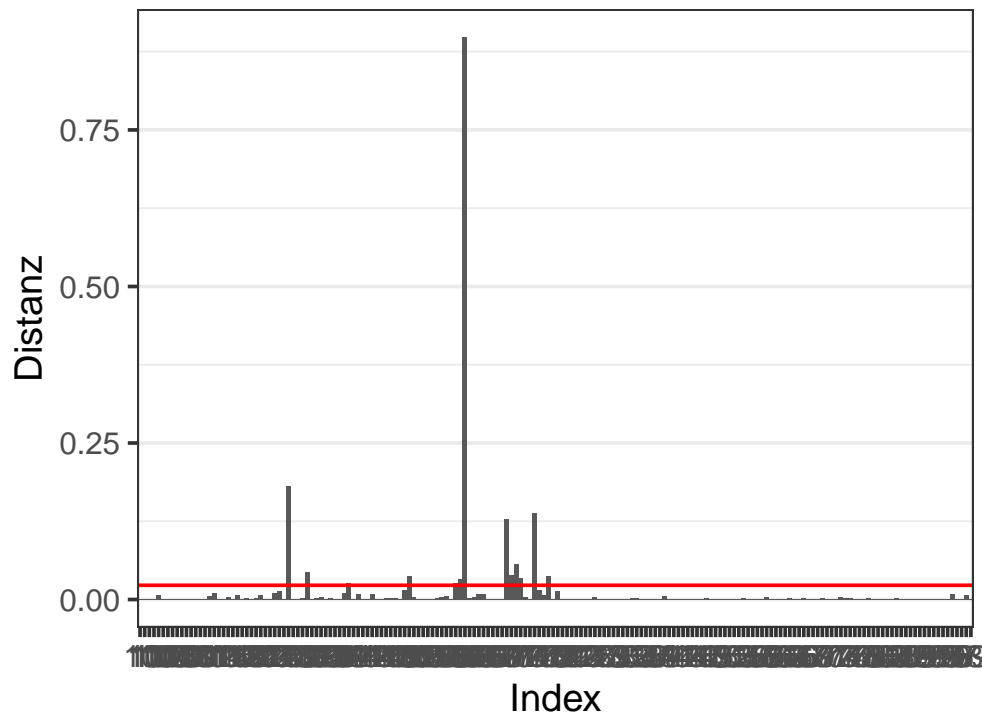
Abbildung 6.15: Betrachtung der Ausreißer nach der Cook'schen Distanz
