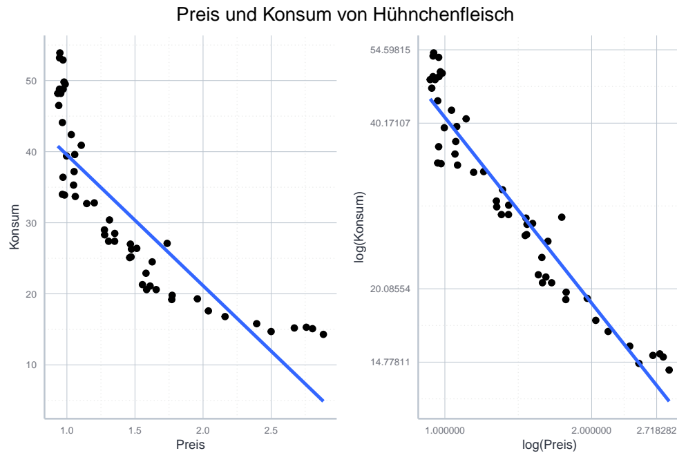
Abbildung 11.22: Nicht-linearer und logarithmierter Zusammenhang zwischen Preis und Konsum von Hühnchenpreis.
