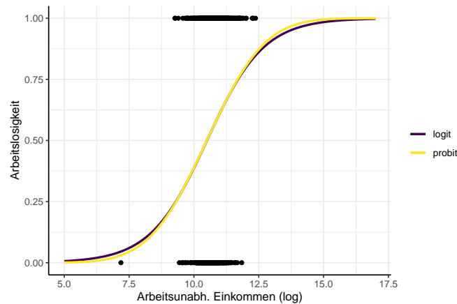
Abbildung 12.3: Vergleich der funktionalen Form bei logit und probit Modellen.
