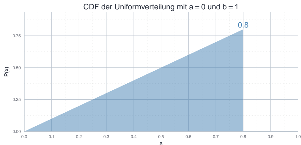
Abbildung 7.13: CDF der Uniformverteilung mit a = 0 und b = 1
