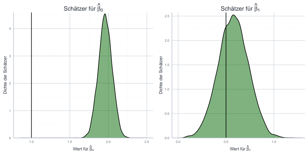
Abbildung 11.12: Folgen der vergessenen Variablen mit Bezug auf Erwartungstreue anhand von Monte Carlo Simulationen.
