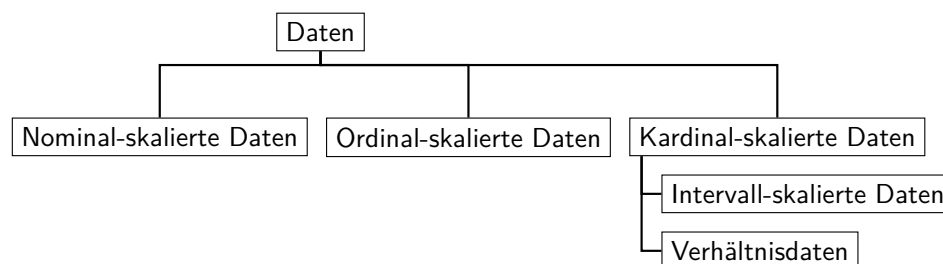
Abbildung 4.2: Skalenniveaus von Daten
