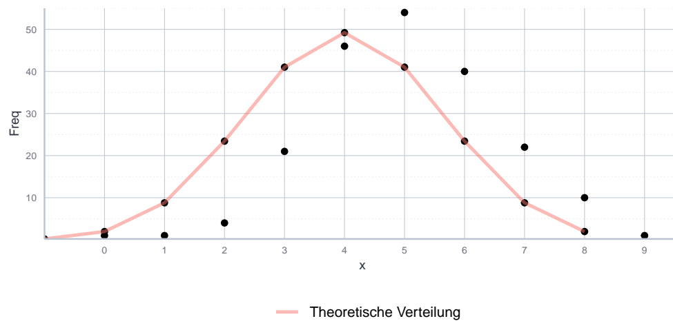
Abbildung 7.6: Vergleich der empirischen Stichprobe und der parametrisierten theoretischen Binomialverteilungsfunktion
