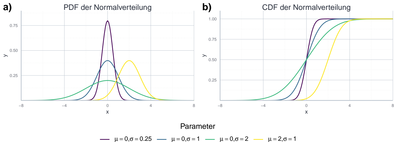
Abbildung 7.14: Vergleich der PDF und CDF der Normalverteilung.
