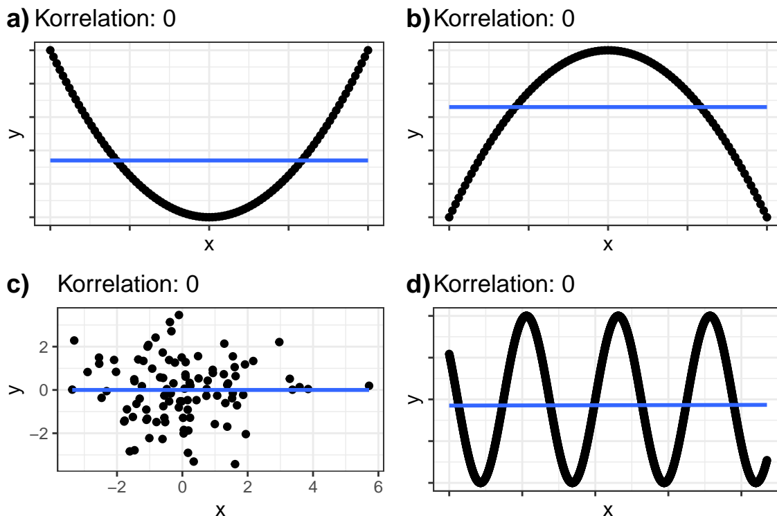
Abbildung 8.1: Unterschiedliche Daten mit gleichen Korrelationswerten.
