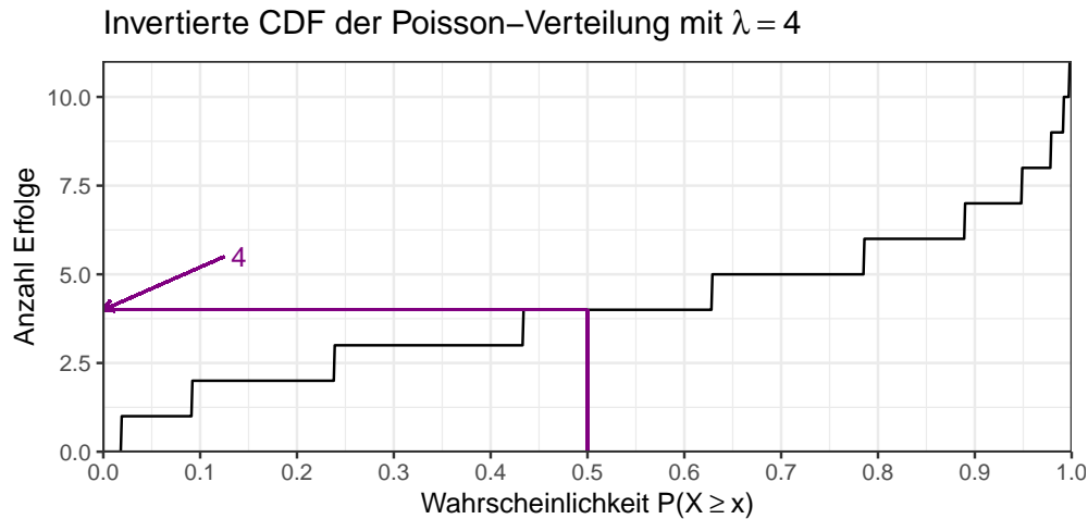
Abbildung 7.10: Invertierte CDF der Poisson-Verteilung mit \lambda = 4
