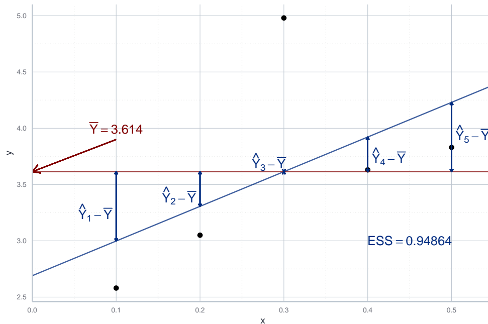
Abbildung 10.5: Variation in der abhängigen Variable, die durch die Regression erklärt wird (ESS).
