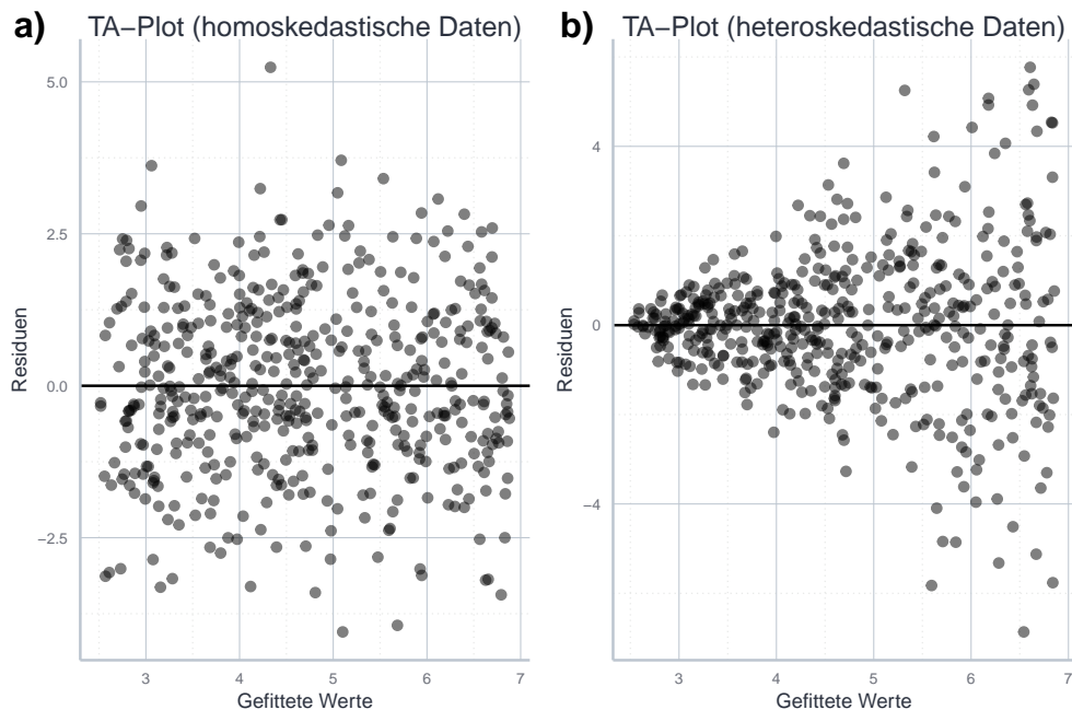
Abbildung 11.7: Graphische Analyse der Homoskedastie.
