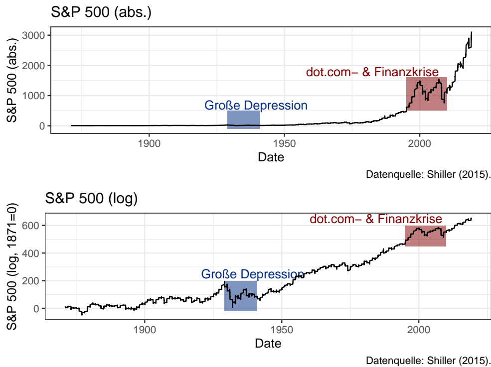
Abbildung 6.3: Vergleich normaler und logarithmierter Darstellung bei Events, die zu sehr unterschiedlichen Zeitpunkten stattgefunden haben
