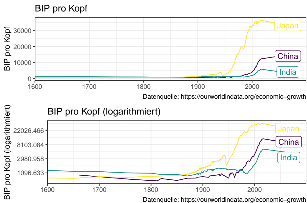
Abbildung 6.2: Vergleich normaler und logarithmierter Darstellung bei langfristiger vergleichender Betrachtung von Wachstumsraten
