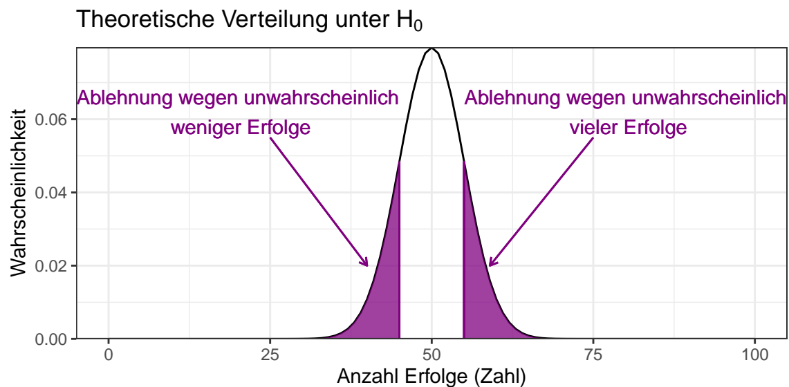
Abbildung 9.2: Verwerfungsbereich der theoretischen Verteilung unter H_0 für \alpha = 0.05 .
