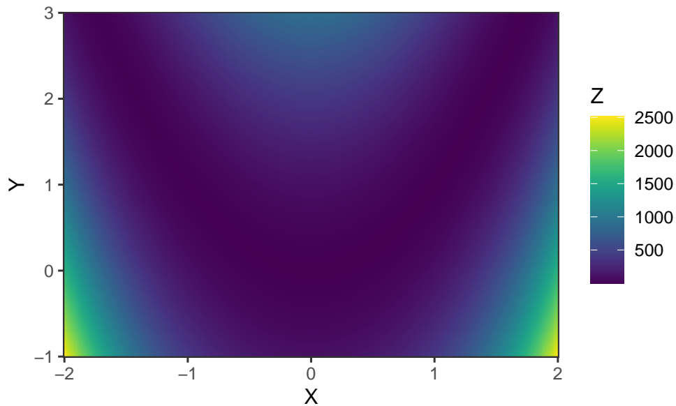
Abbildung 6.7: Darstellung einer Funktion als Heatmap
