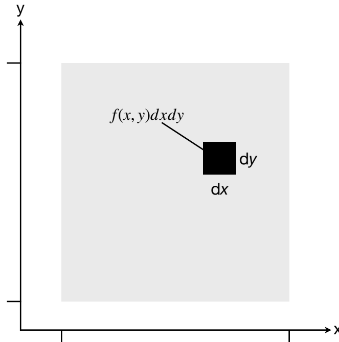
Abbildung 7.16: Gemeinsame Verteilung zweier stetiger ZV. Die Wahrscheinlichkeit eines Events korrespondiert zur Fläche.
