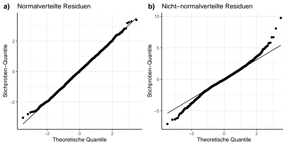
Abbildung 11.23: Q-Q-Plot zur Überprüfung der Residuen.
