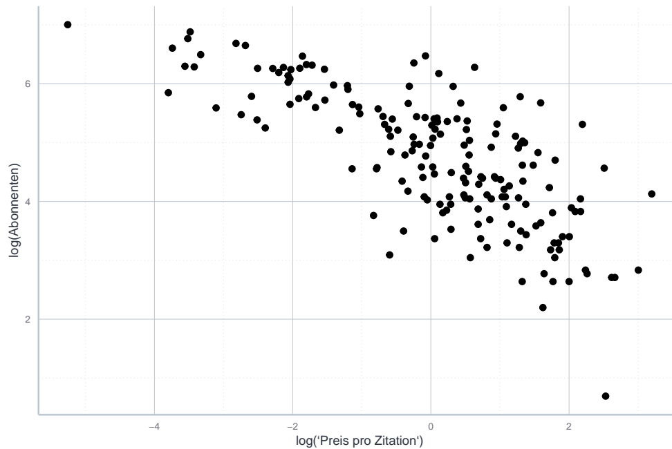
Abbildung 11.21: Logarithmierter Zusammenhang zwischen Abonnenten und Preis pro Zitation.
