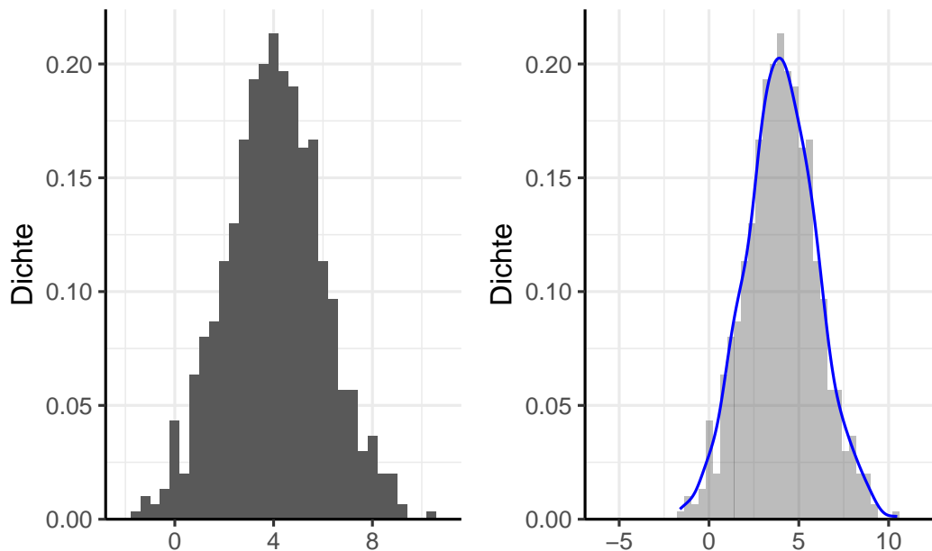
Abbildung 6.8: Stichprobe (linker Graph) und Stichprobe mit empirischer Dichtefunktion (rechter Graph)
