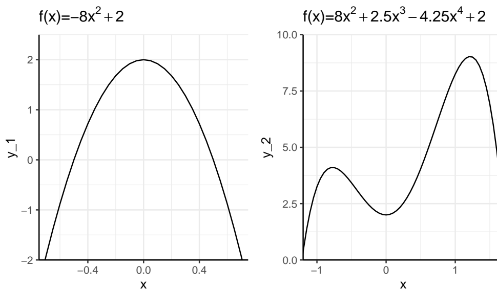
Abbildung 6.5: Beispiel für die Gefahr auf einem lokalen Extremum hängen zu bleiben (rechter Graph).
