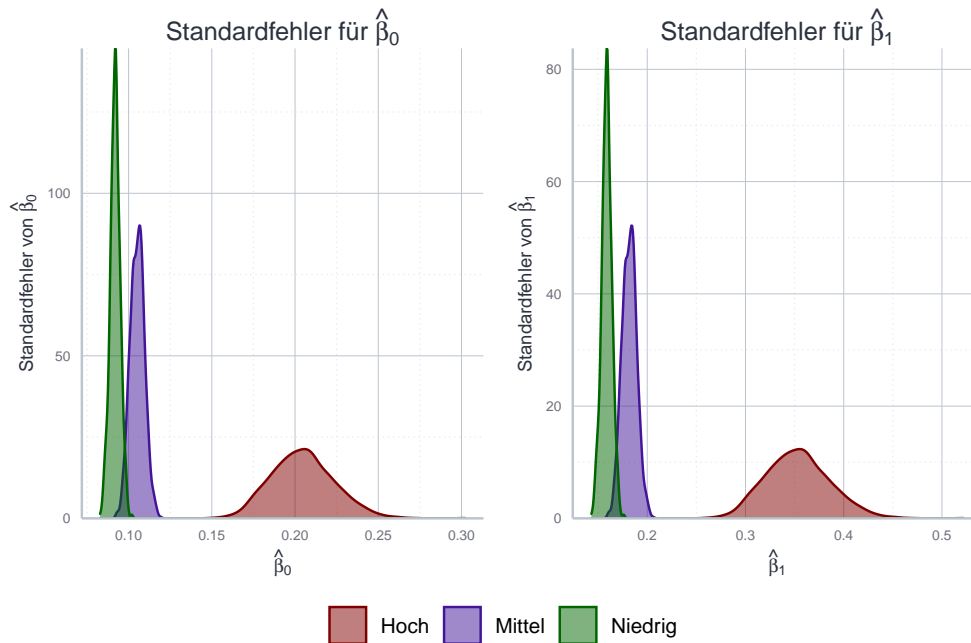
Abbildung 11.9: Folgen der Autokorrelation mit Bezug auf Standardfehler anhand von Monte Carlo Simulationen.
