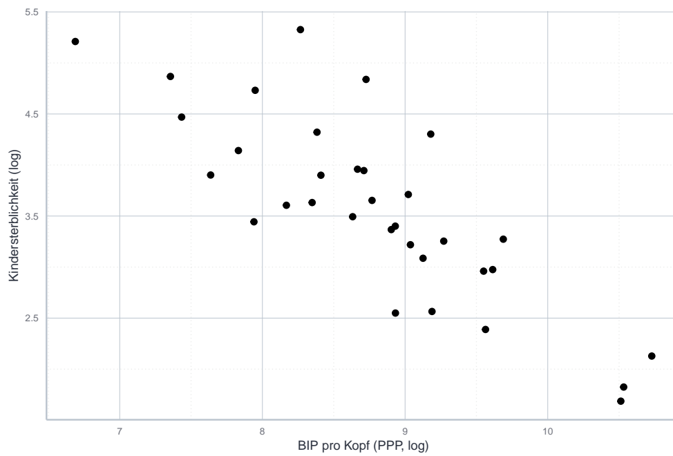
Abbildung 11.15: Logarithmierter Zusammenhang zwischen BIP und Kindersterblichkeit.
