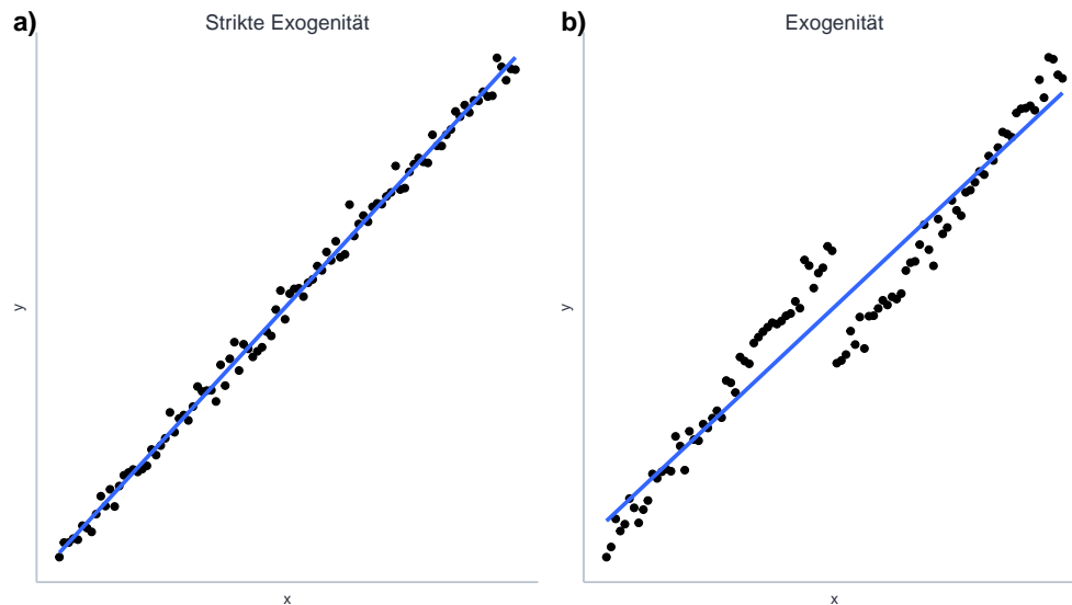
Abbildung 11.2: Exogenität und strikte Exogenität.
