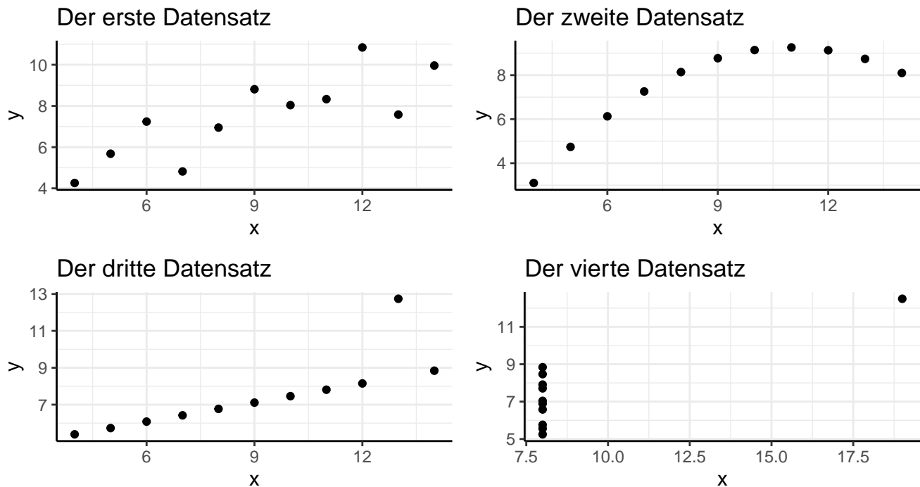
Abbildung 8.2: Unterschiedliche Daten mit gleichen Korrelationswerten.
