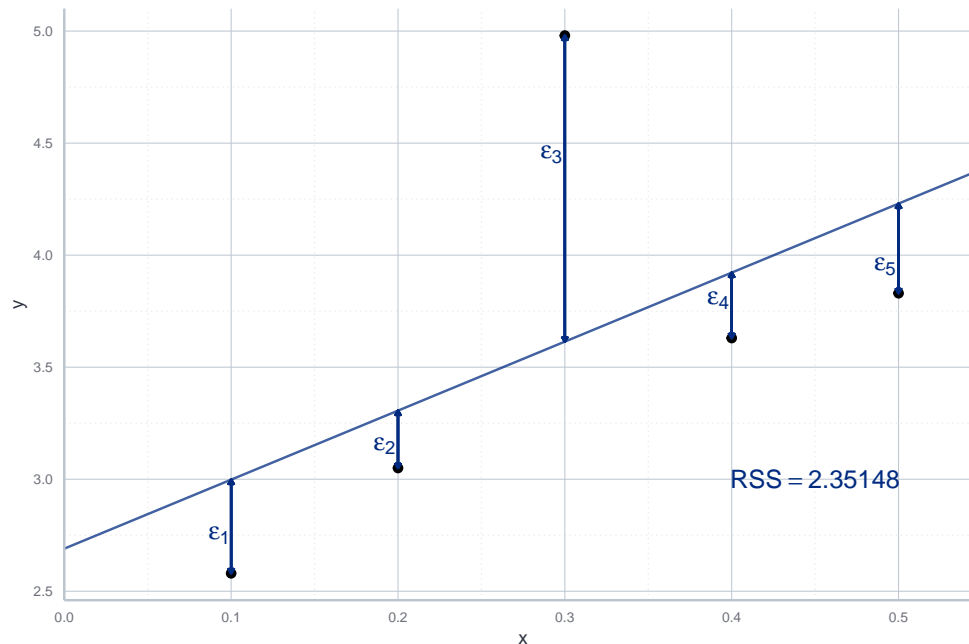
Abbildung 10.4: Abweichungen der geschätzten Werte und den tatsächlichen Werten, i.e. den Residuen (RSS).
