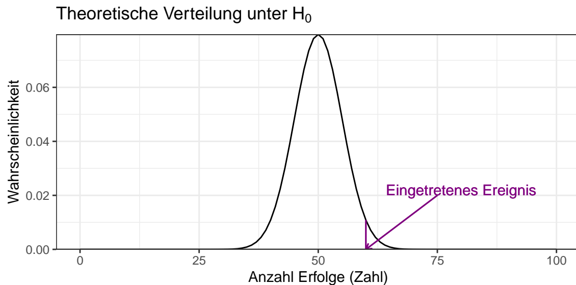
Abbildung 9.1: Vergleich unseres eingetretenen Ereignisses mit der theoretischen Verteilung unter H_0 .
