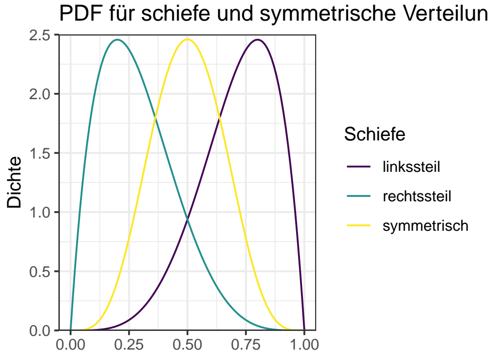
Abbildung 6.12: Beispiele für Verteilungen mit unterschiedlichen Schiefen
